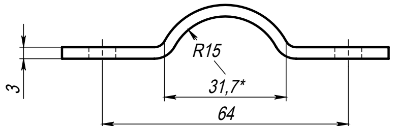
Поз. 1 (Полухомут)
