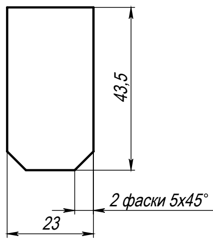
Поз. 3 (Ребро)
